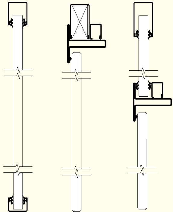
Vertikalschnitt. Festwand.
